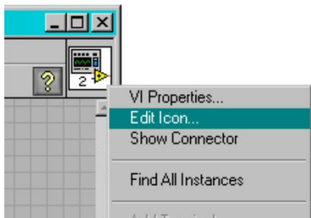
Рисунок 22 Выбор режима
