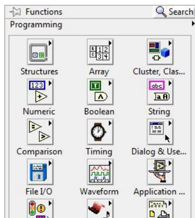
Рисунок 13 – Палитра функций
