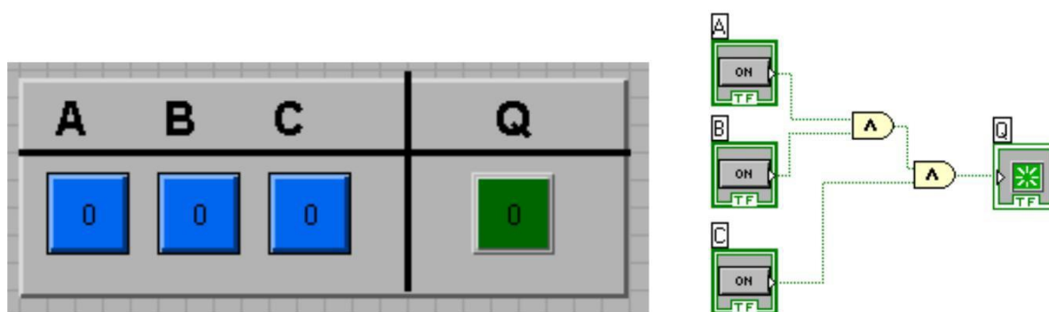
Рисунок 20 - Модель логического элемента И с тремя входами
