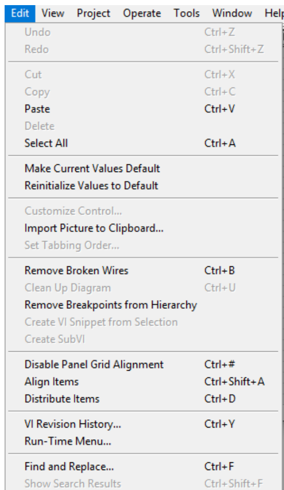
Рисунок 6 – Вкладка редактировать.
