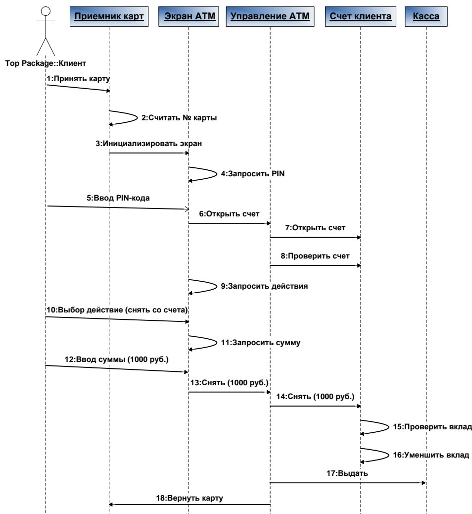
Рисунок 41 - Диаграмма последовательностей
