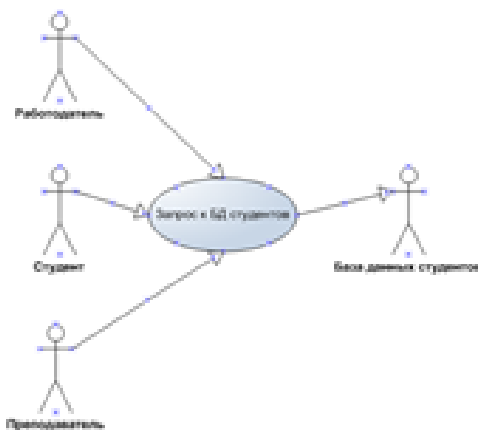
Рисунок 46 – UML-диаграмма
