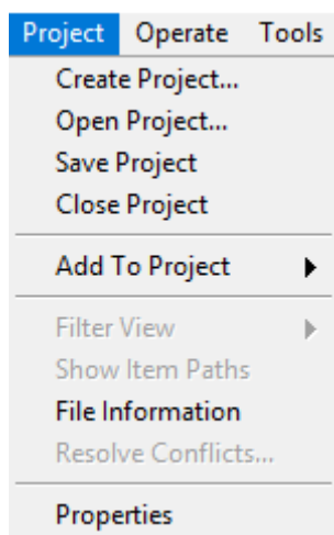
Рисунок 4 – Вкладка проект.
