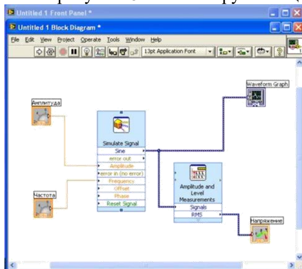
Рисунок 18 – Блок схема.
