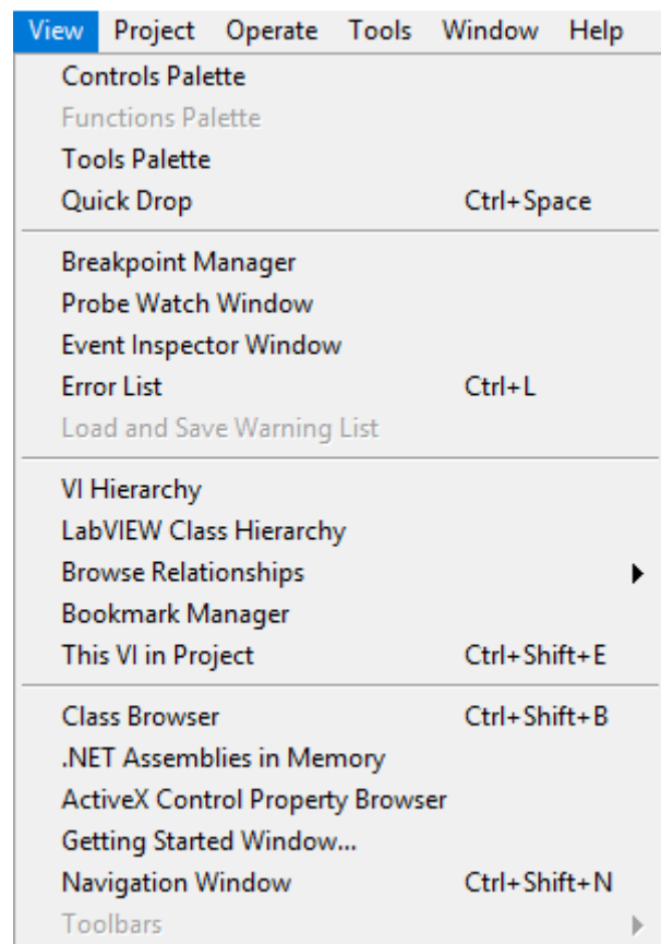
Рисунок 7 – Вкладка посмотреть.
