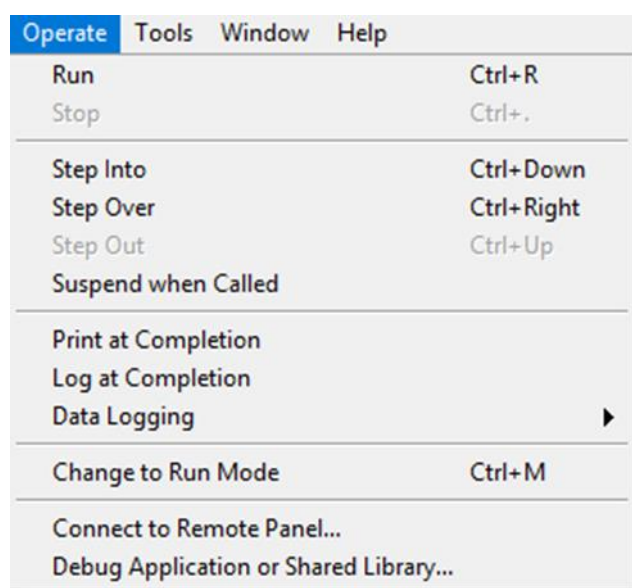
Рисунок 5- Вкладка действия.
