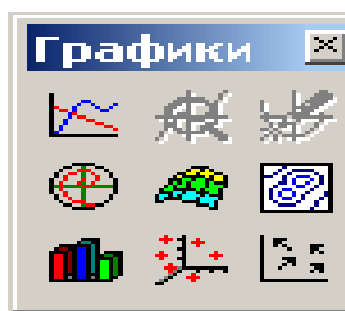
Рисунок 18 – Панель графиков
