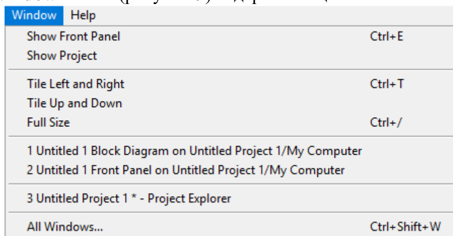
Рисунок 9 – Вкладка окно.
