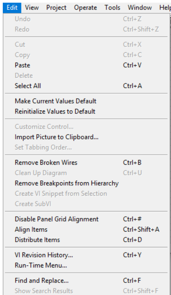
Рисунок 6 – Вкладка редактировать.
