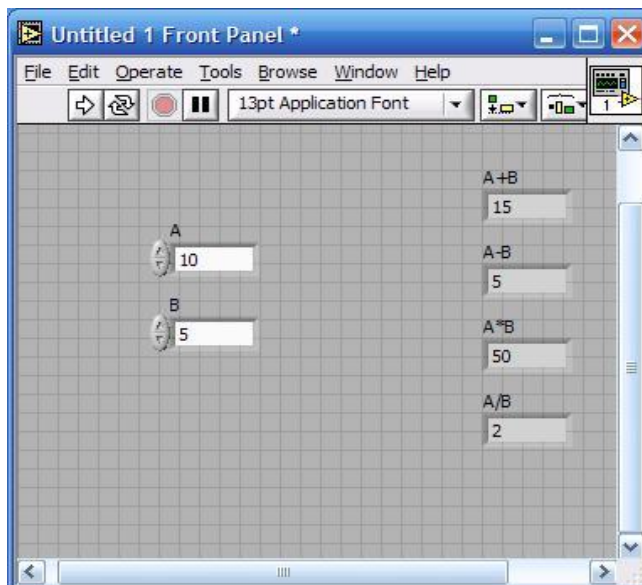
Рисунок 14 –Лицевая панель
