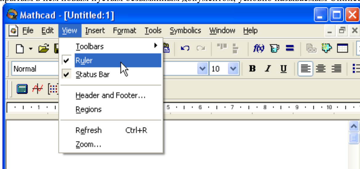
Рисунок 7 – Вызов линейки
