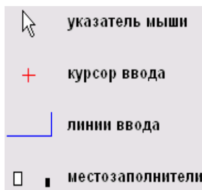
Рисунок 8 – Интерфейс редактирования
