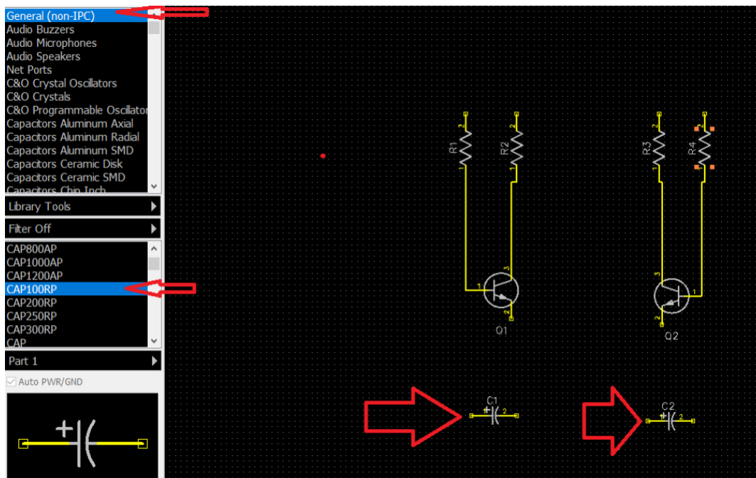
Рисунок 8. 20 – Добавление CAP 100RP
