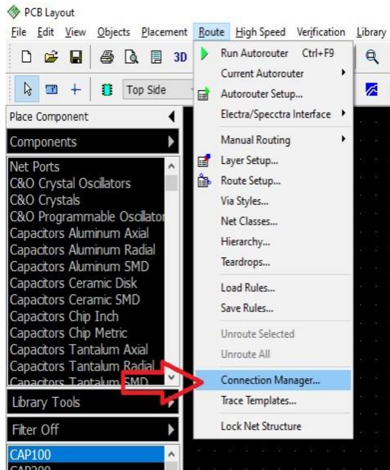
Рисунок 8.31 – Создание связей вручную
