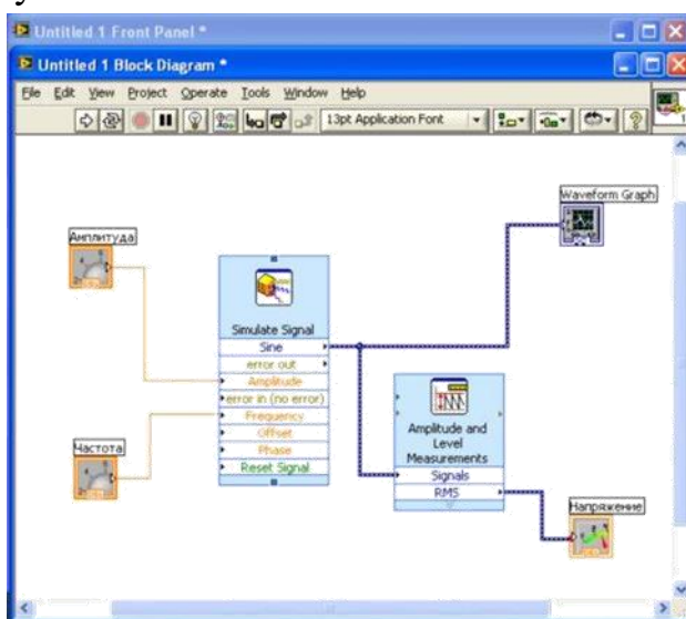
Рисунок 8.17 – Блок схема.
