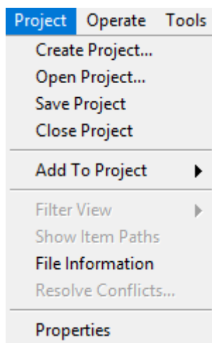
Рисунок 4 – Вкладка проект.
