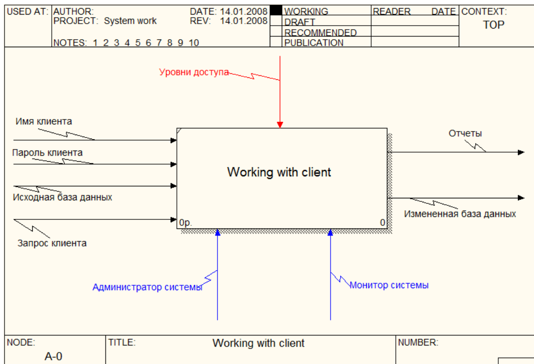
Рисунок 12 - Контекстная диаграмма в BPwin
