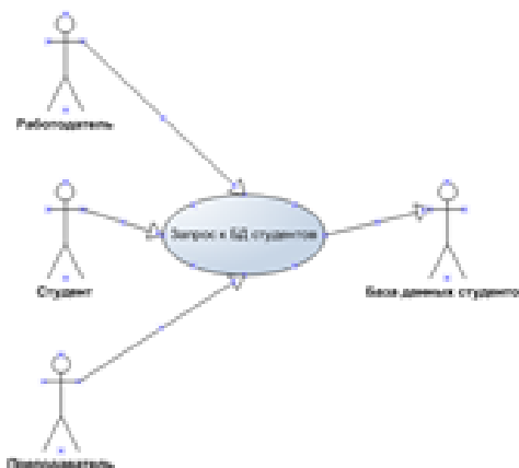
Рисунок 46 – UML-диаграмма
