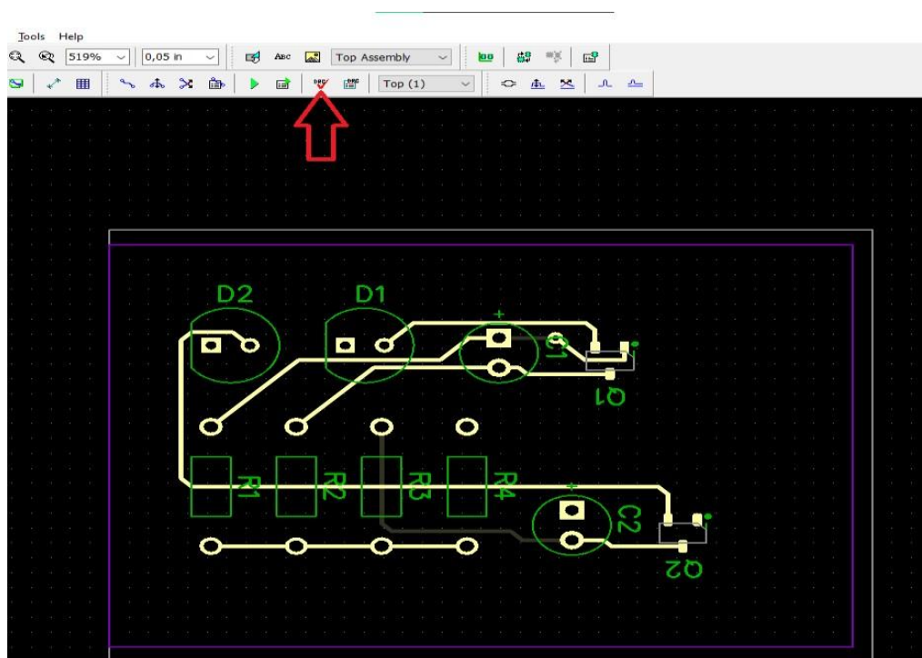
Рисунок 8.37 – Автоматическая проверка DRC
