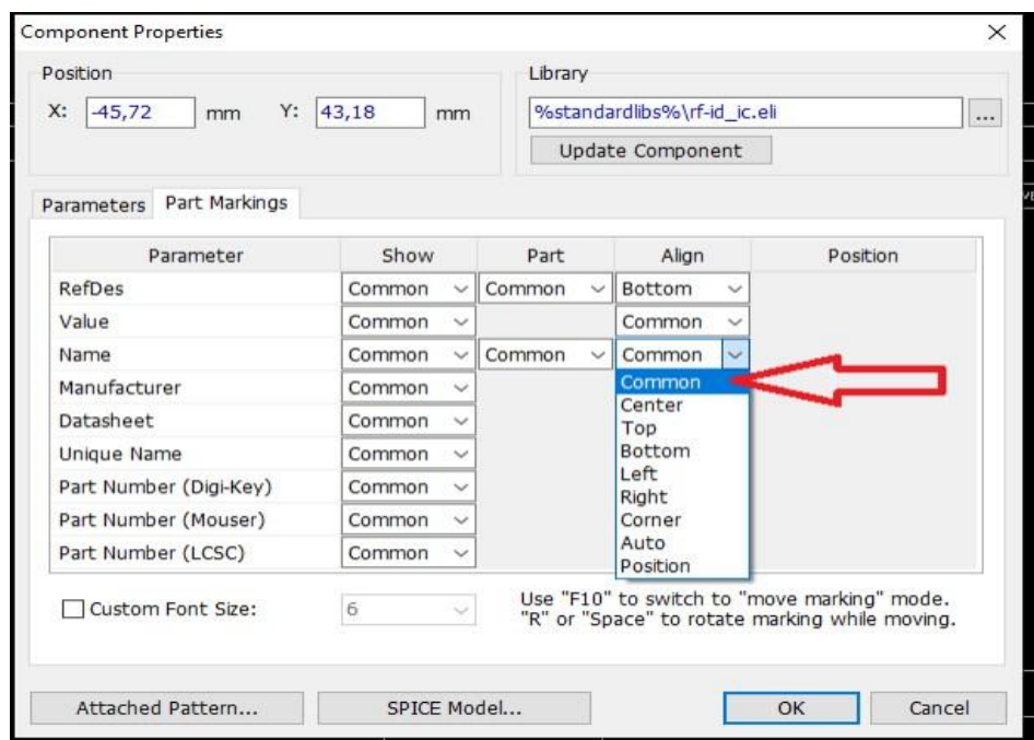
Рисунок 8.17 – Пункт настройки по названию маркировки компонента
