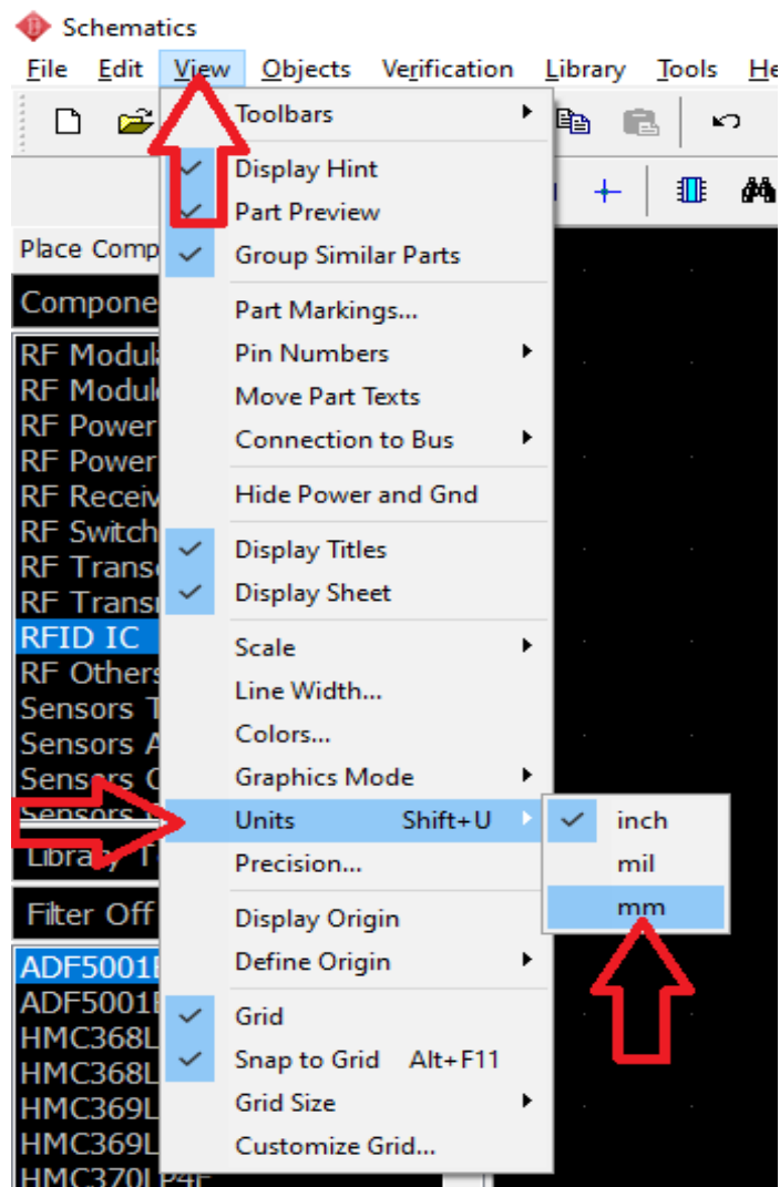
Рисунок 8.12 – Пункт изменения единиц измерения
