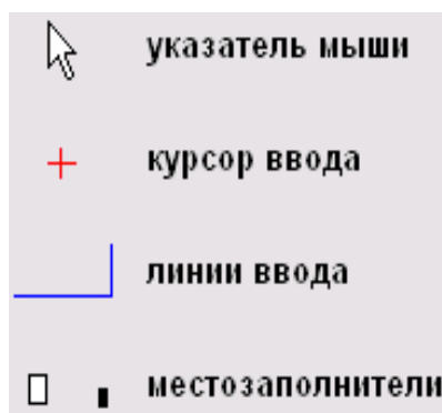
Рисунок 8 – Интерфейс редактирования
