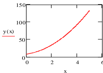
Рисунок 19 – Построение графика
