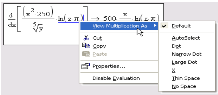
Рисунок 2 – Контекстное меню
