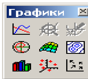
Рисунок 18 – Панель графиков
